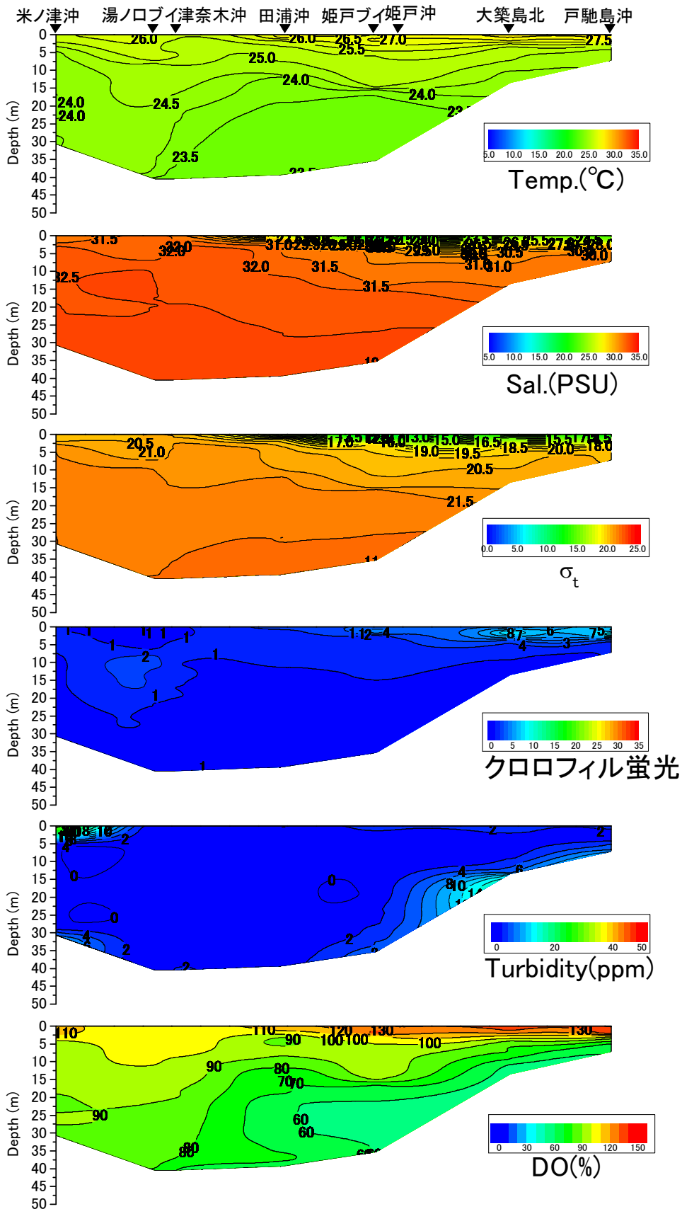
戸馳島沖から米ノ津沖の水温(°C)、塩分、密度( \sigma_t )、クロロフィル蛍光強度、濁度、溶存酸素飽和度(DO%)の鉛直面図(東町漁業協同組合の調査による) (2014年8月7日)
